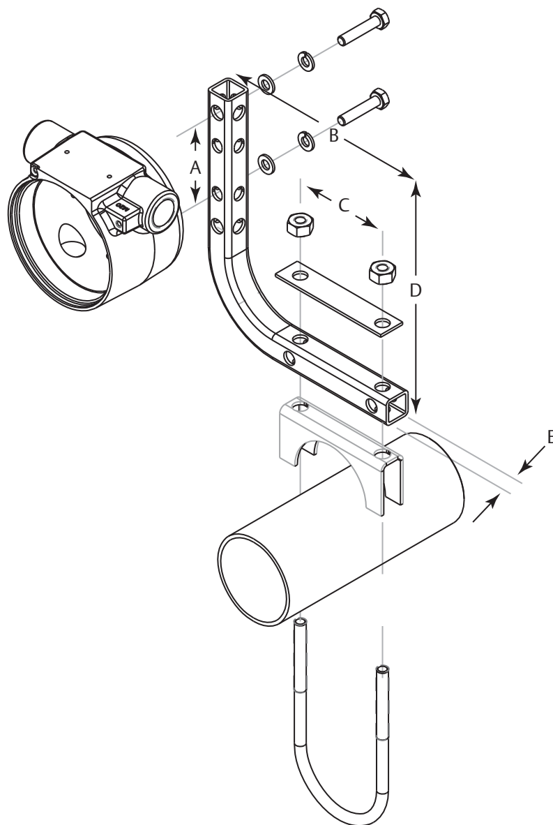
选项编码为 B5 的安装架
