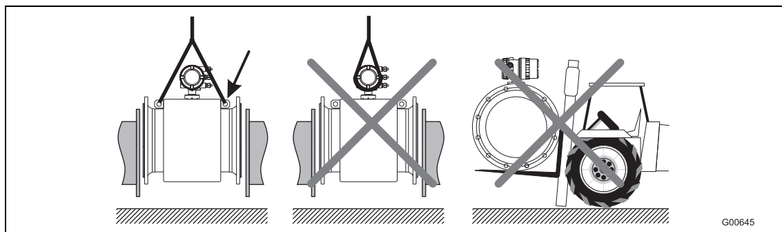
图 6：DN 400 以上尺寸法兰连接设备的运输
